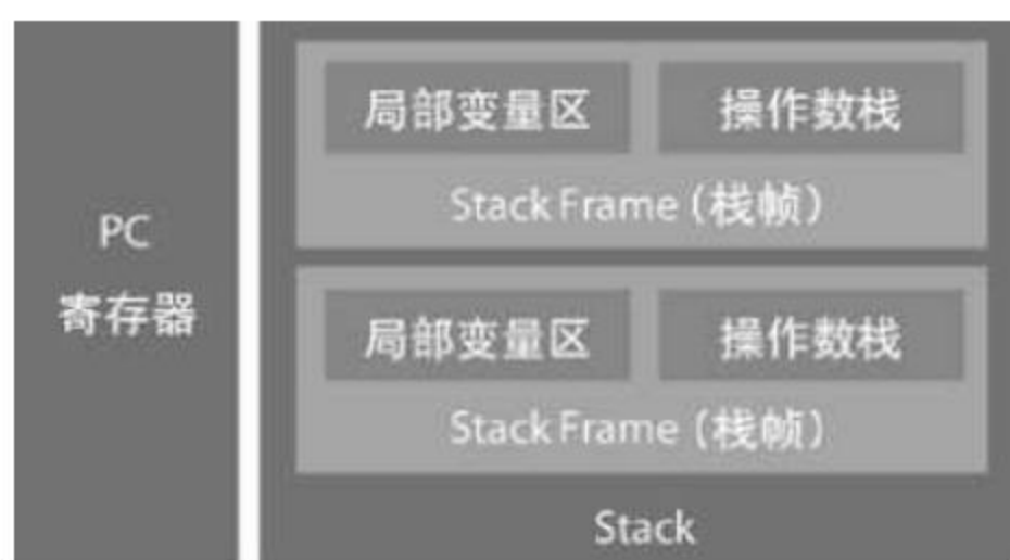
图 3.5 Sun JDK 基于栈的体系结构
