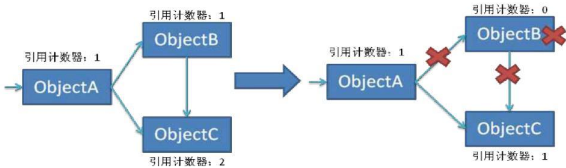
图 3.9 引用计数收集器
