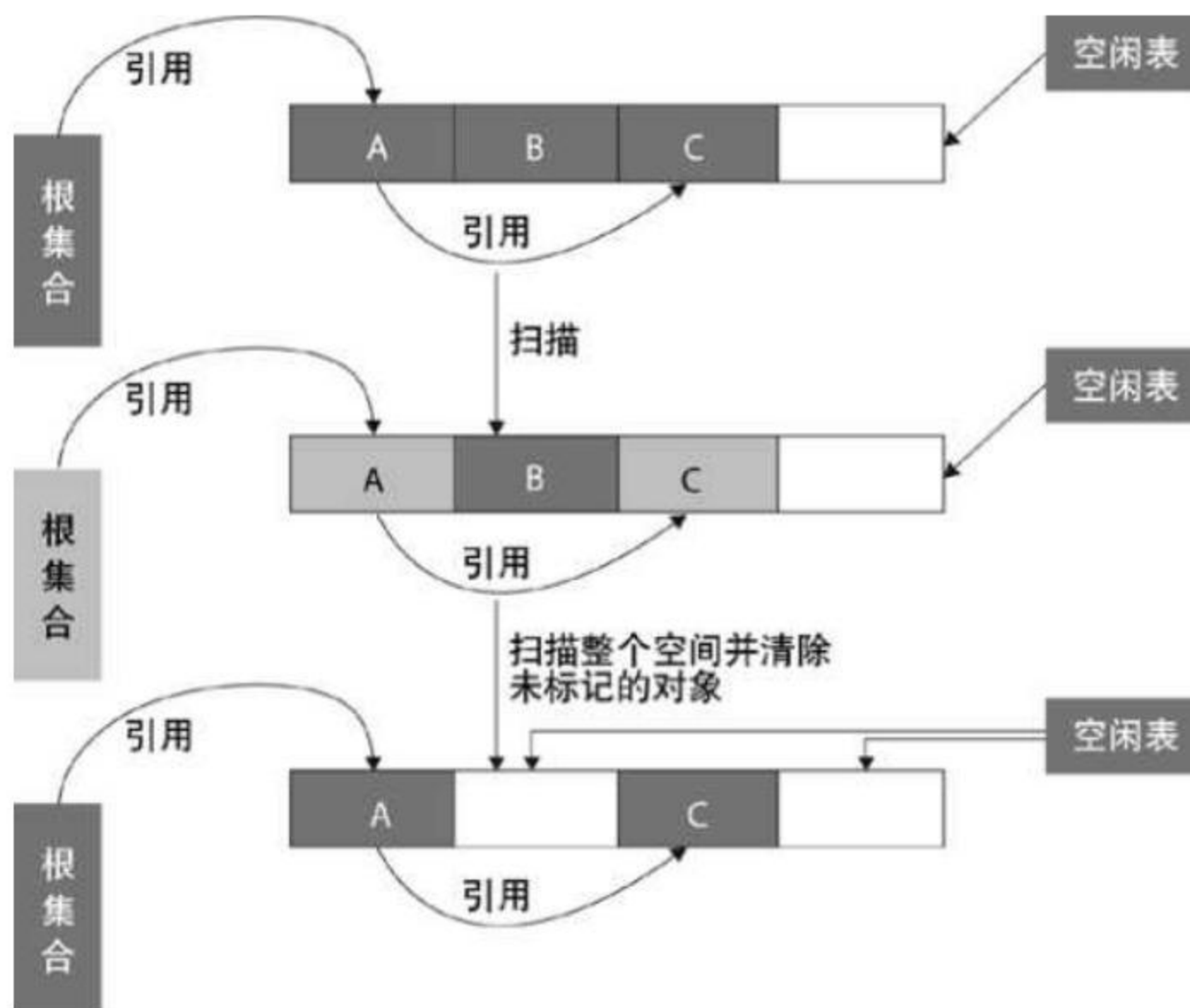
图 3.11 标记-清除算法
