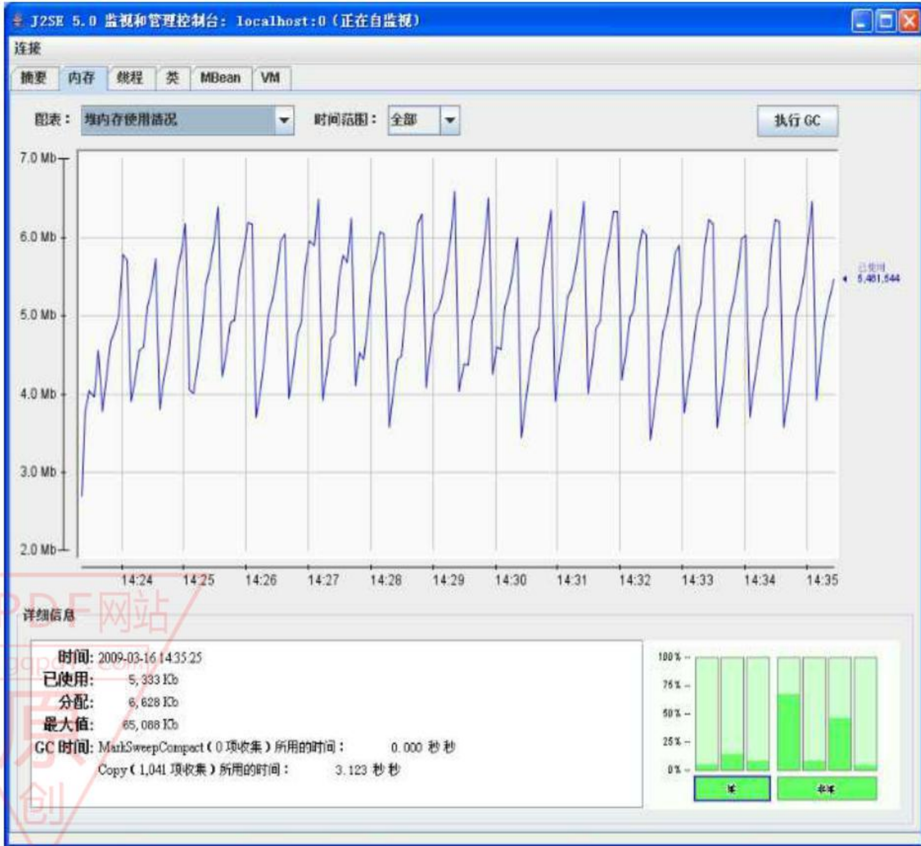
图 3.18 JConsole 运行效果
