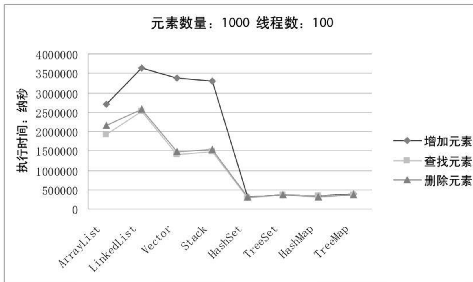
图 4.13 线程数：100，元素数量：1000 时的运行结果对比
