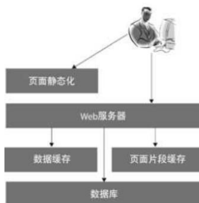
图 7.7 缓存的使用示例
