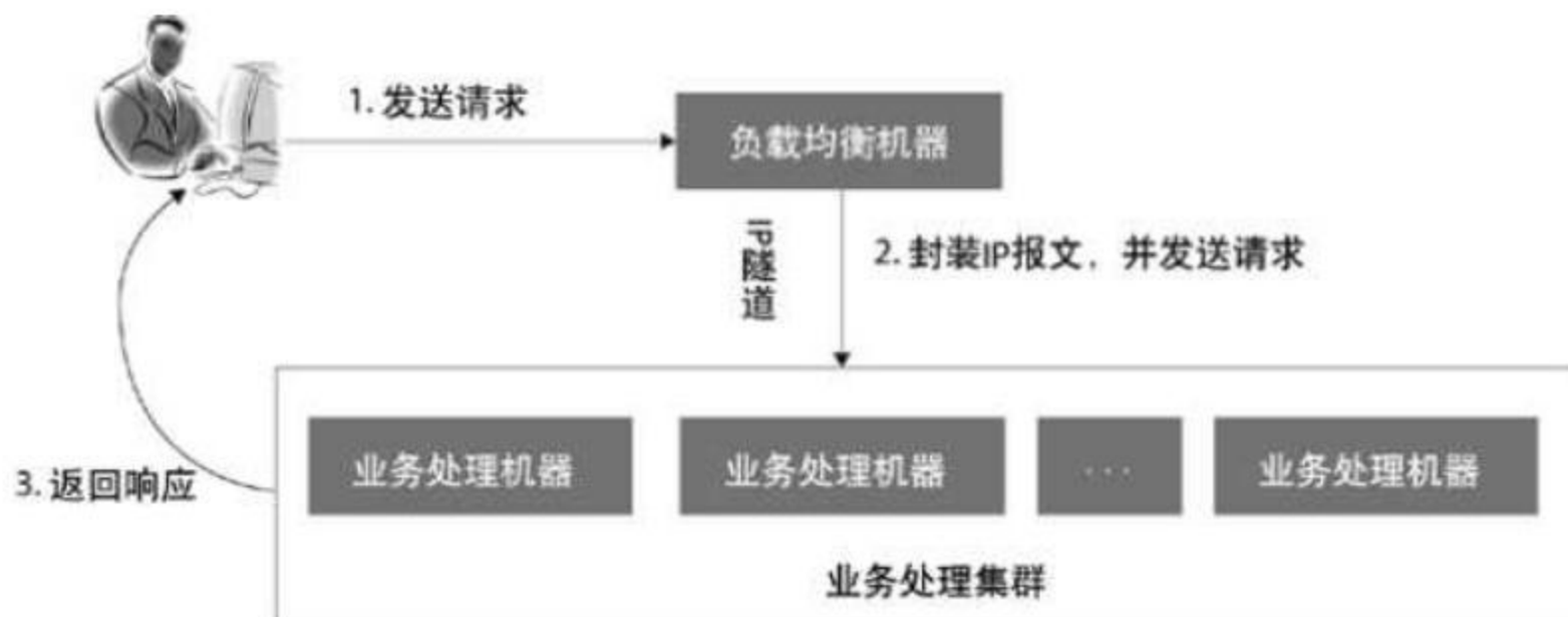
图 6.3 IP Tunneling 方式时的响应返回
