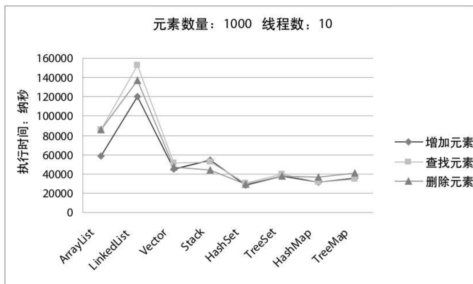
图 4.11 线程数：10，元素数量：1000 时的运行结果对比
