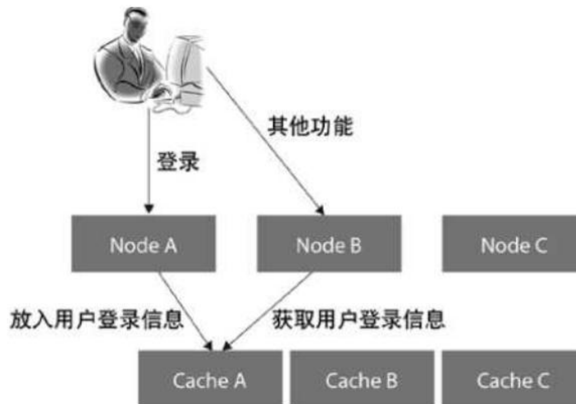
图 7.2 基于分布式缓存实现缓存中的状态一致
