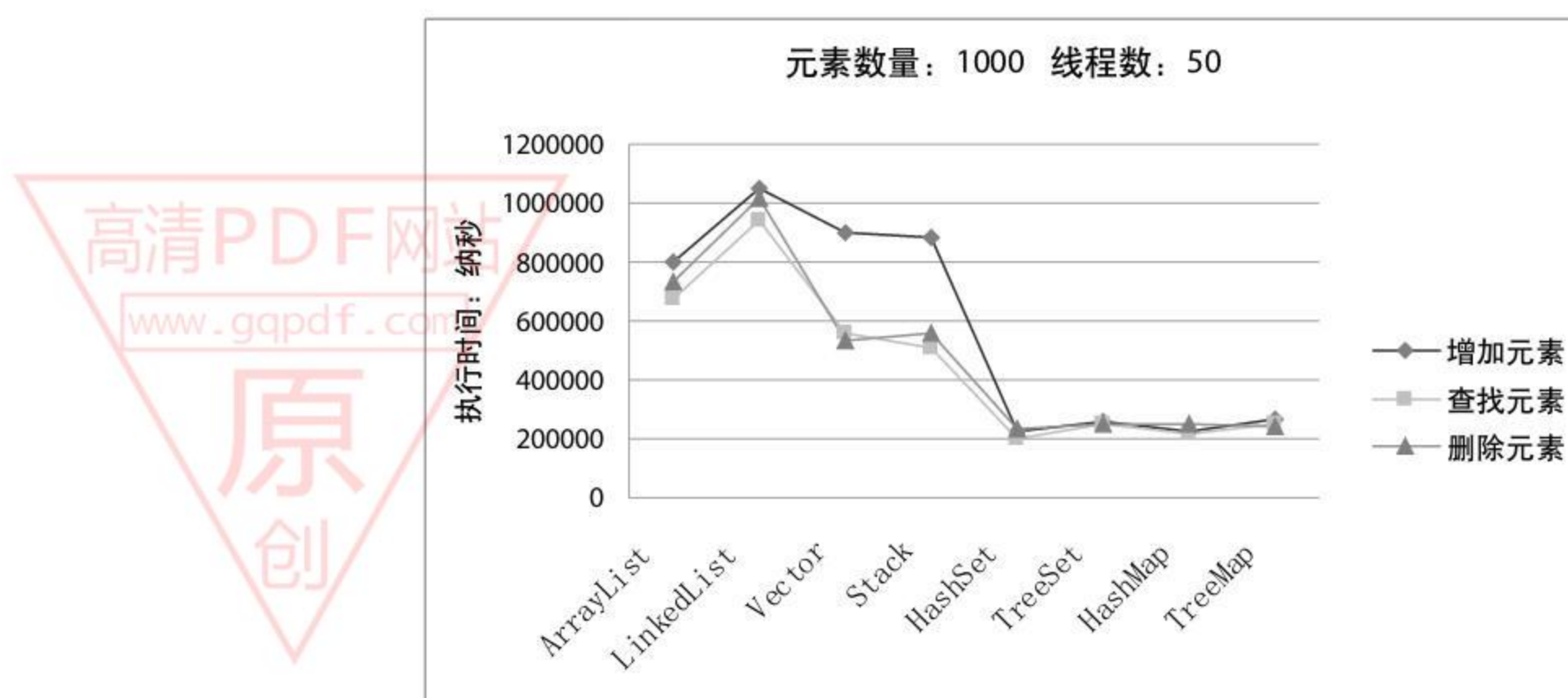
图 4.12 线程数: 50, 元素数量: 1000 时的运行结果对比
