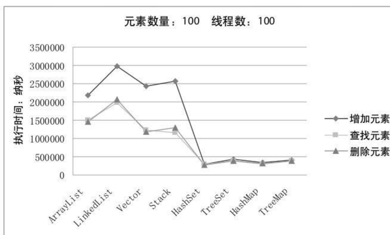
图 4.10 线程数: 100, 元素数量: 100 时的运行结果对比
