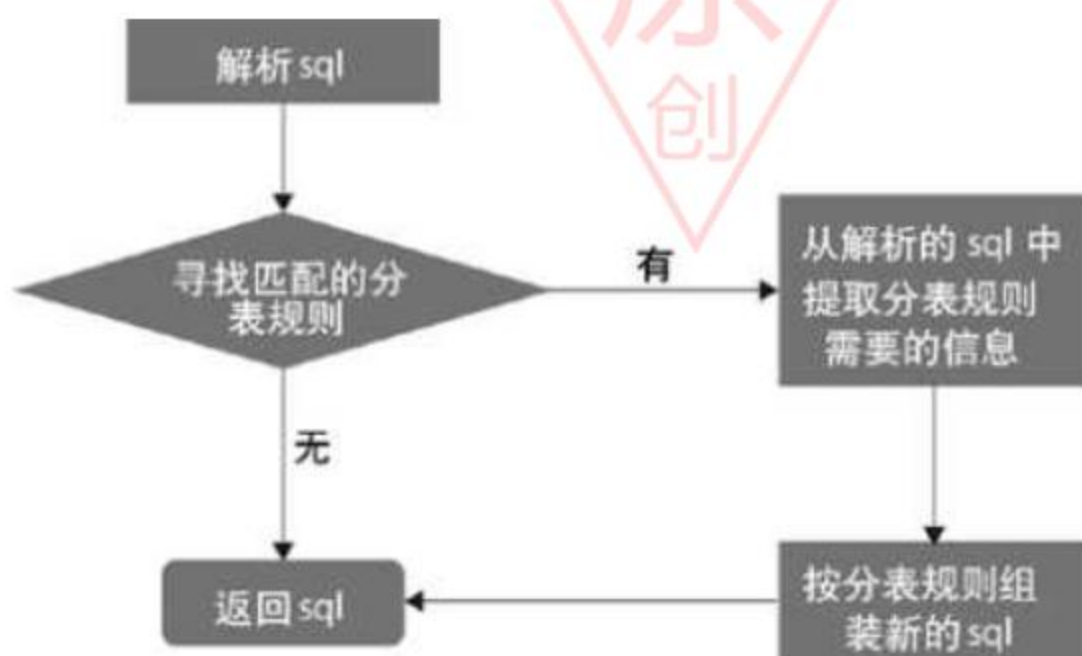
图 7.11 DAL 的执行过程
