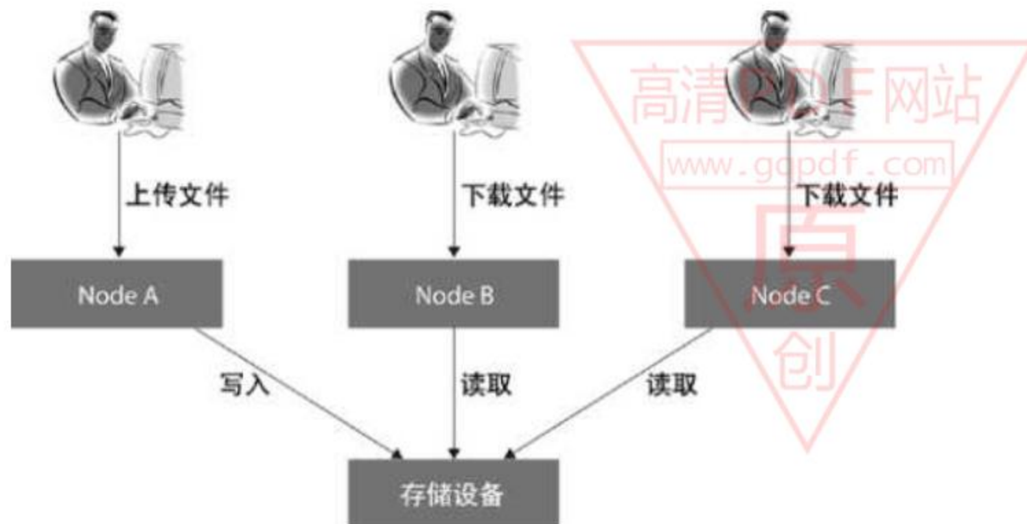
图 7.4 DAS 方式示例
