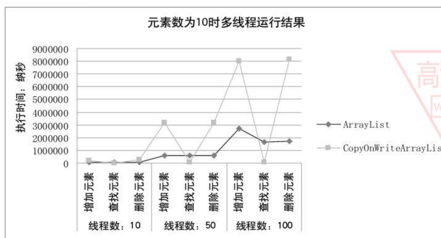
图 4.23 多线程下，元素数为 10 时 CopyOnWriteArrayList 和 ArrayList 的对比
