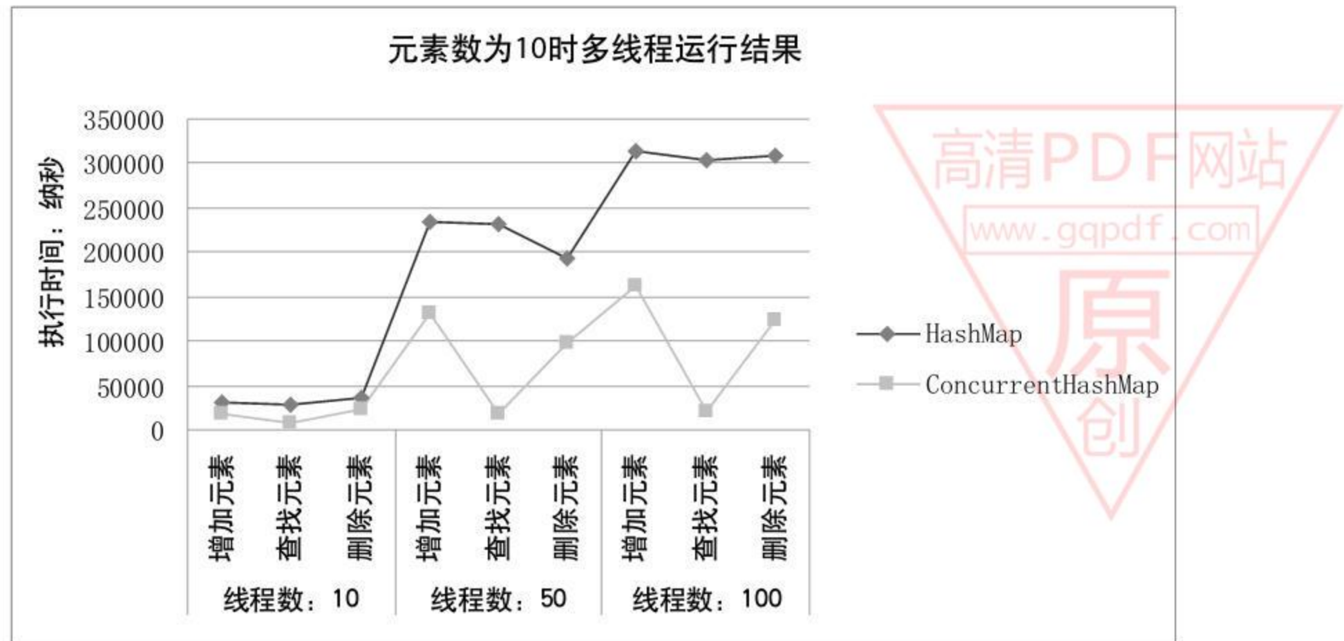
图 4.18 多线程场景，元素数为 10 时 ConcurrentHashMap 和 HashMap 运行结果的对比
