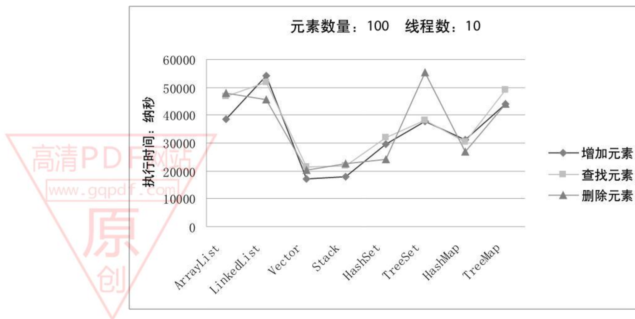
图 4.8 线程数：10，元素数量：100 时的运行结果对比
