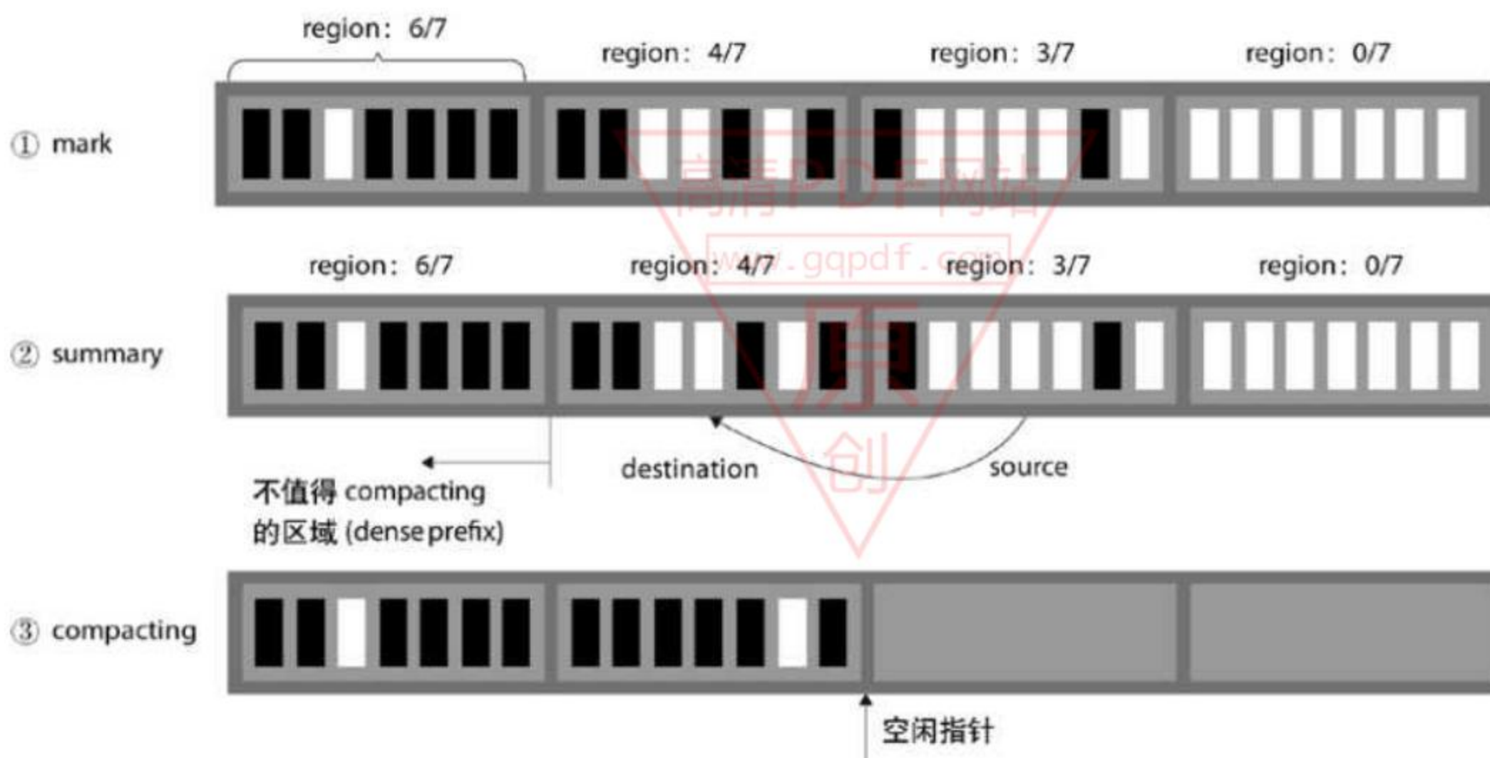
图 3.15 并行 GC 执行过程
