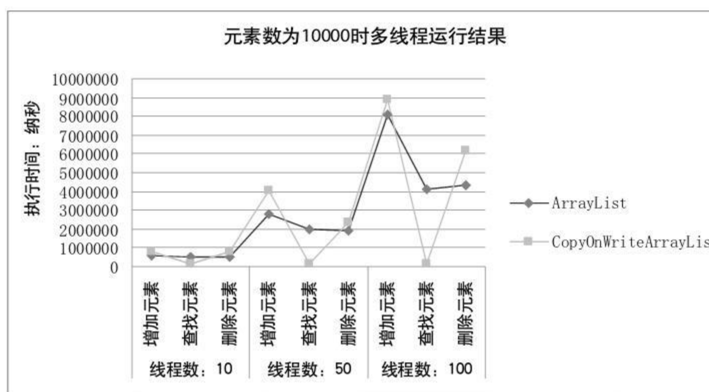
图 4.26 多线程下，元素数为 10000 时 CopyOnWriteArrayLis 和 ArrayList 的对比
