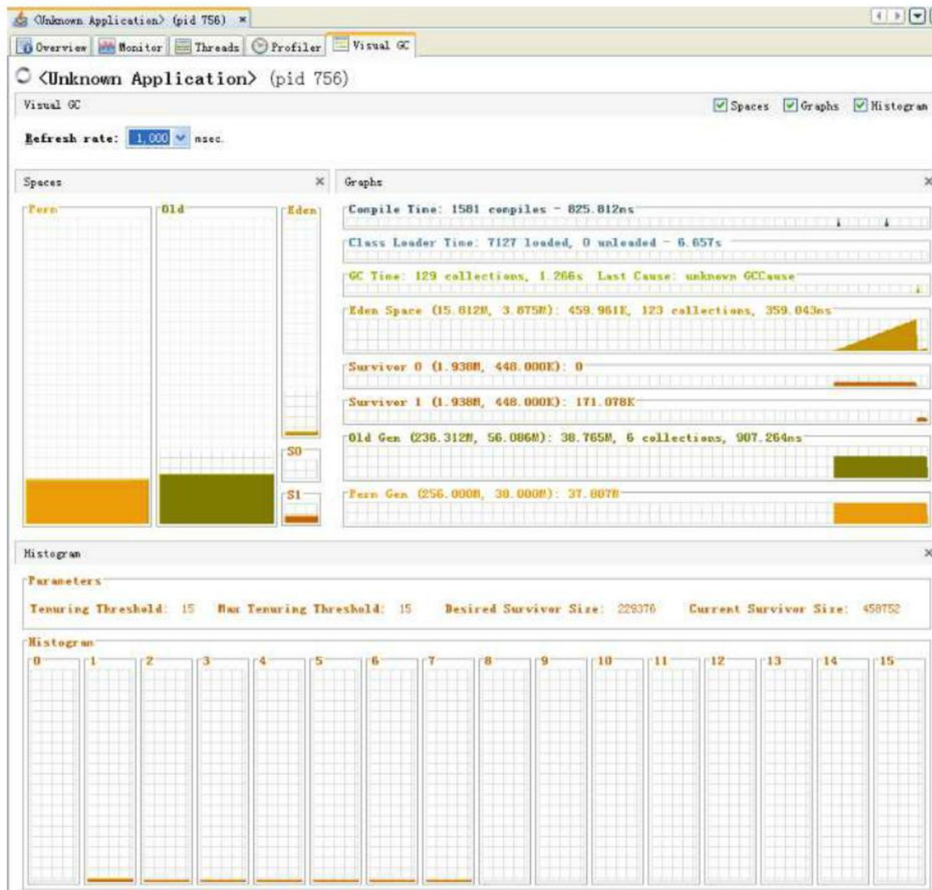
图 3.19 VisualGC 运行效果
