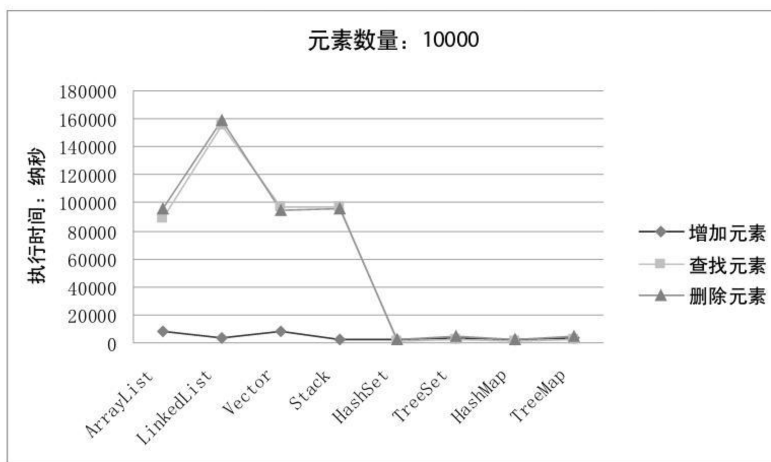
图 4.4 单线程下元素数量为 10000 时的运行结果对比
