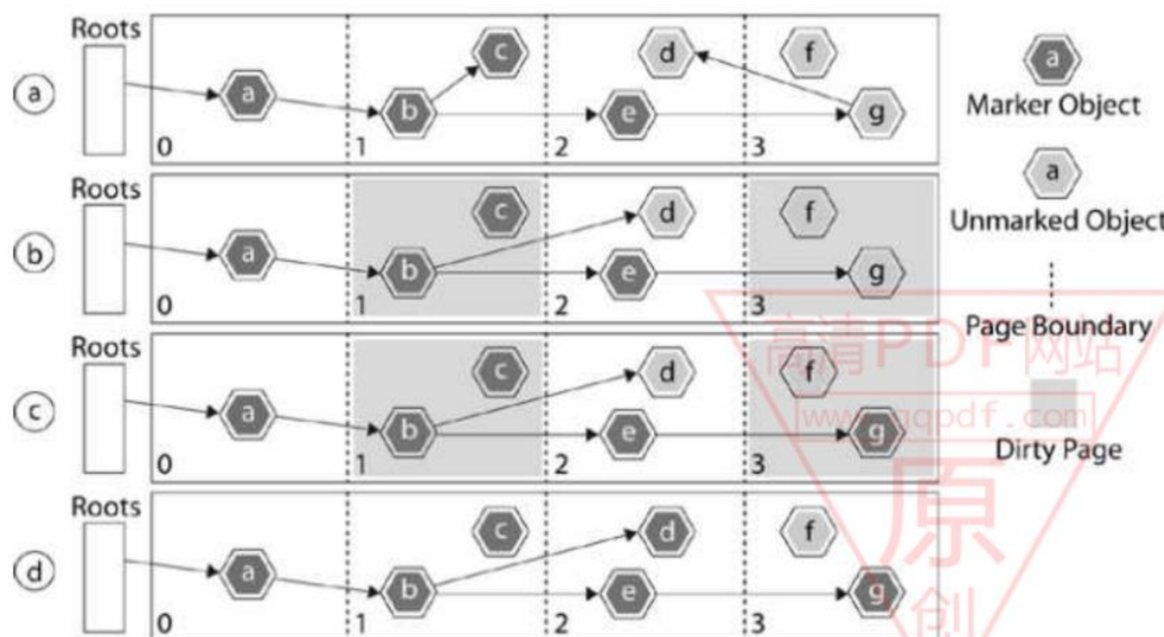
图 3.16 CMS GC 时浮动垃圾产生的示例
