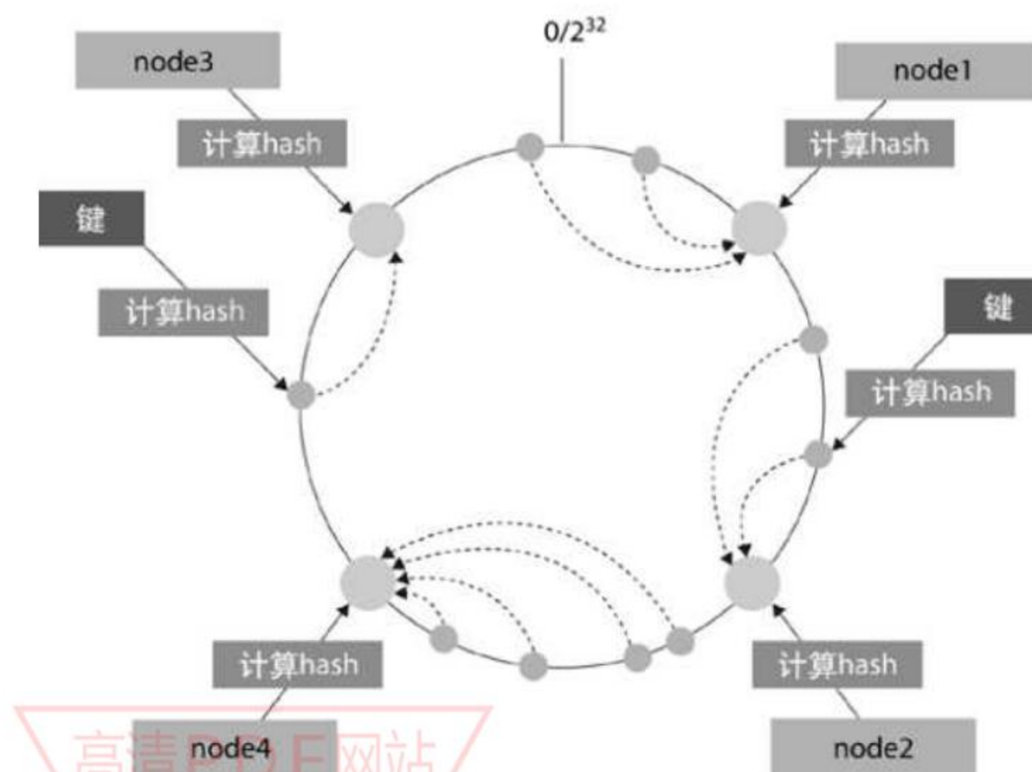
图 7.3 一致性 hash 算法图示
