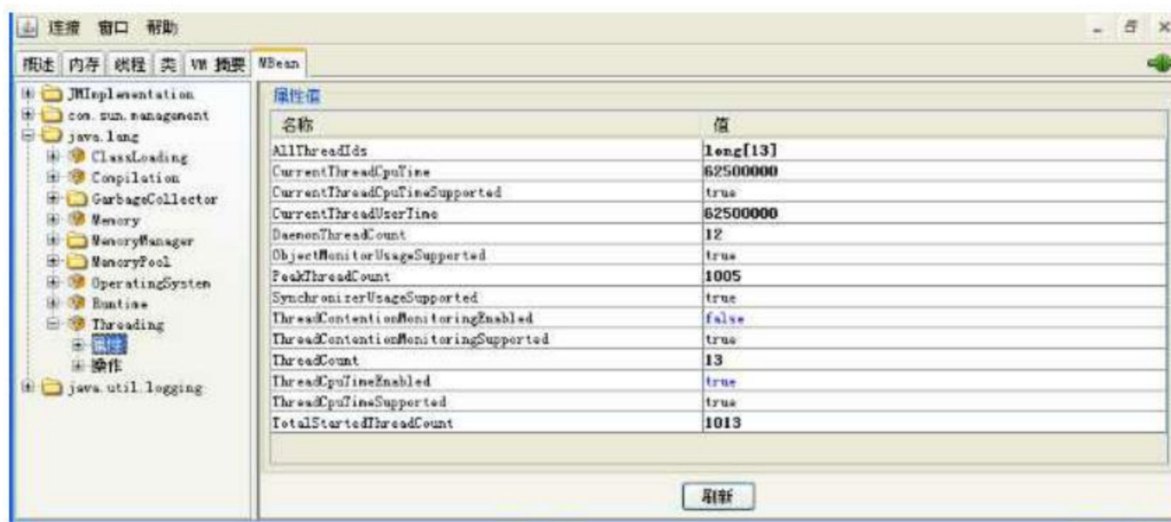
图 3.27 ThreadXMBean 查看线程状态
