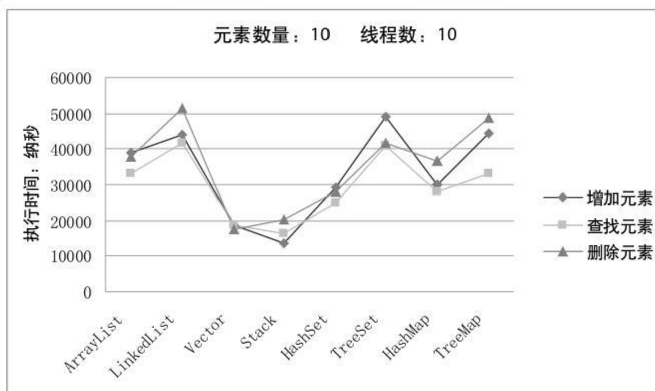
图 4.5 线程数及元素数量均为 10 时的运行结果对比
