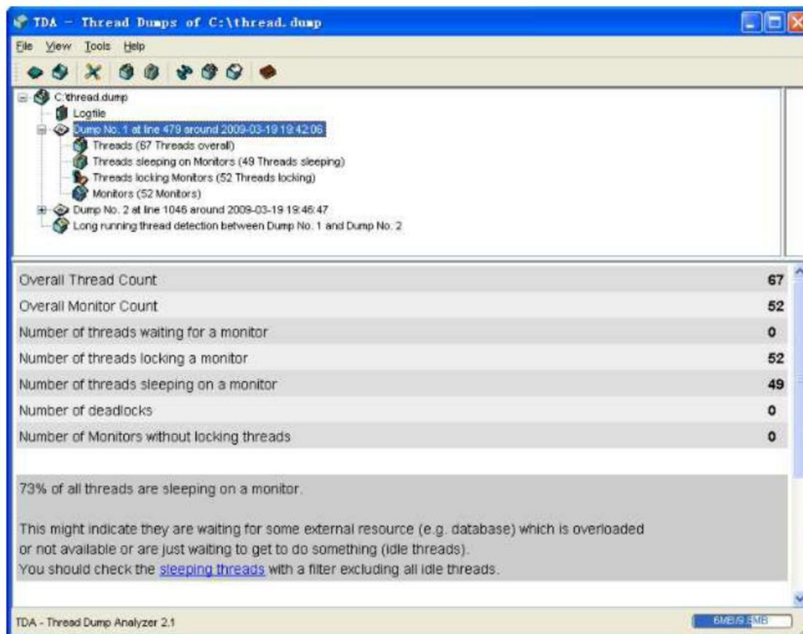
图 3.28 TDA 查看线程状态
