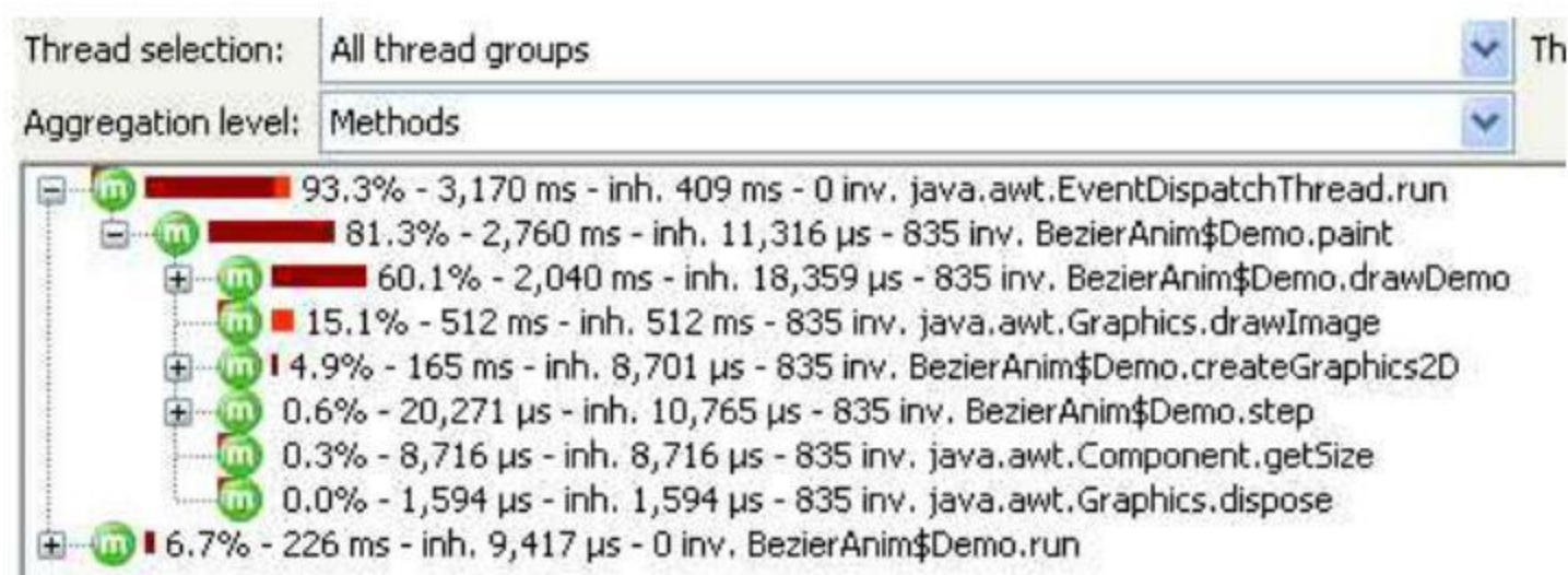
图 5.14 JProfiler 分析程序执行速度
