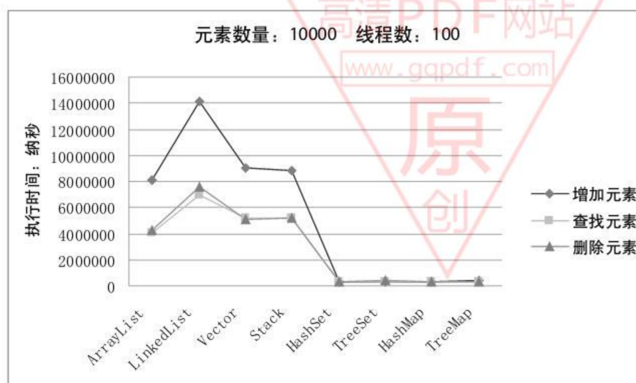
图 4.16 线程数：100，元素数量：10000 时的运行结果对比
