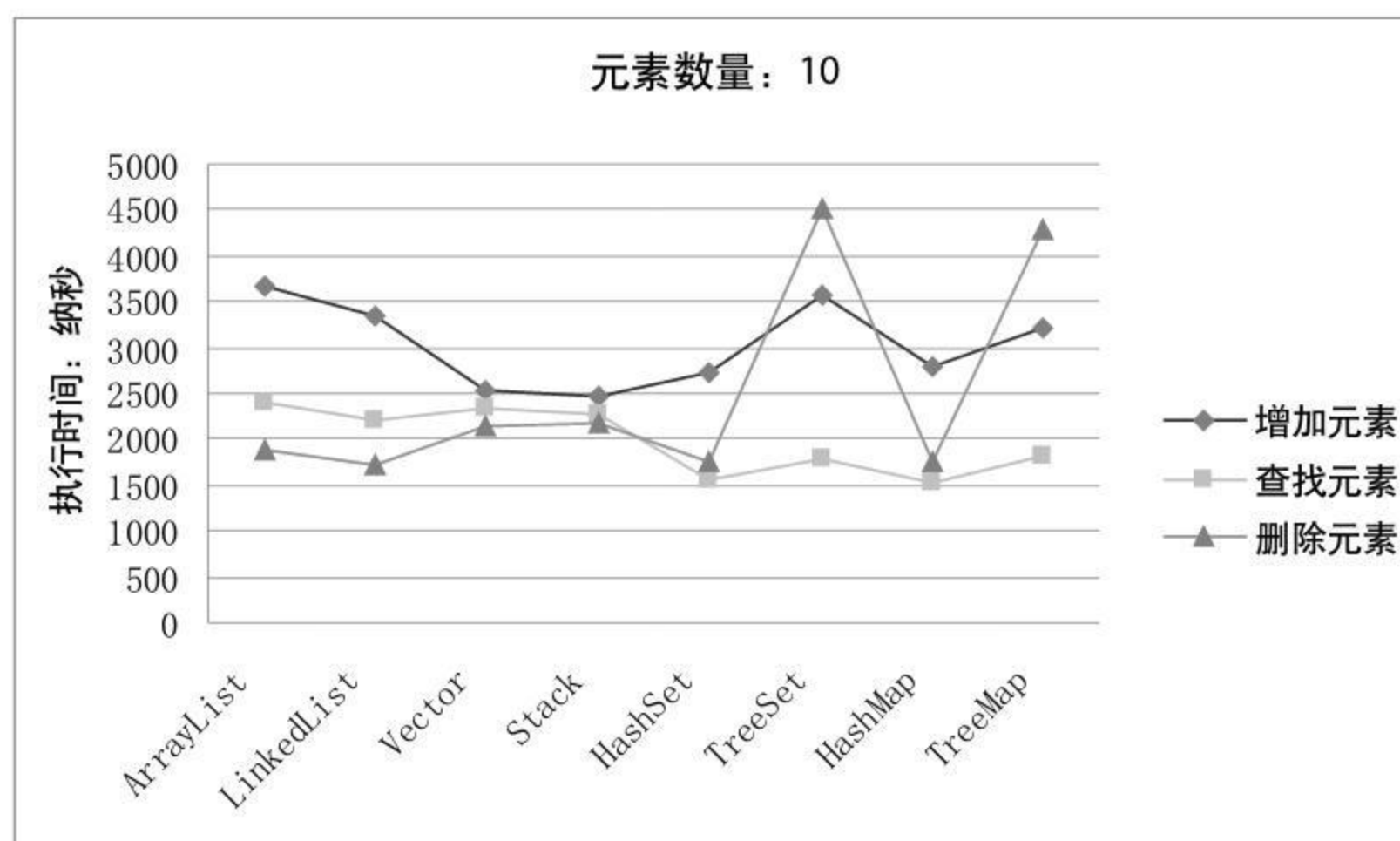
图 4.1 单线程下元素数量为 10 时的运行结果对比
