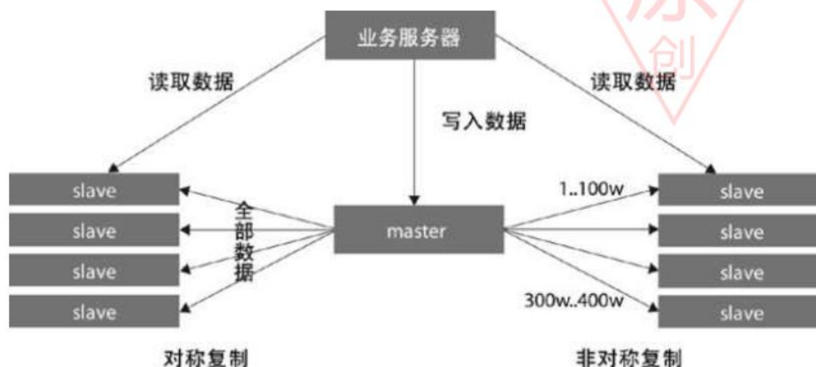
图 7.12 读写分离后的系统结构
