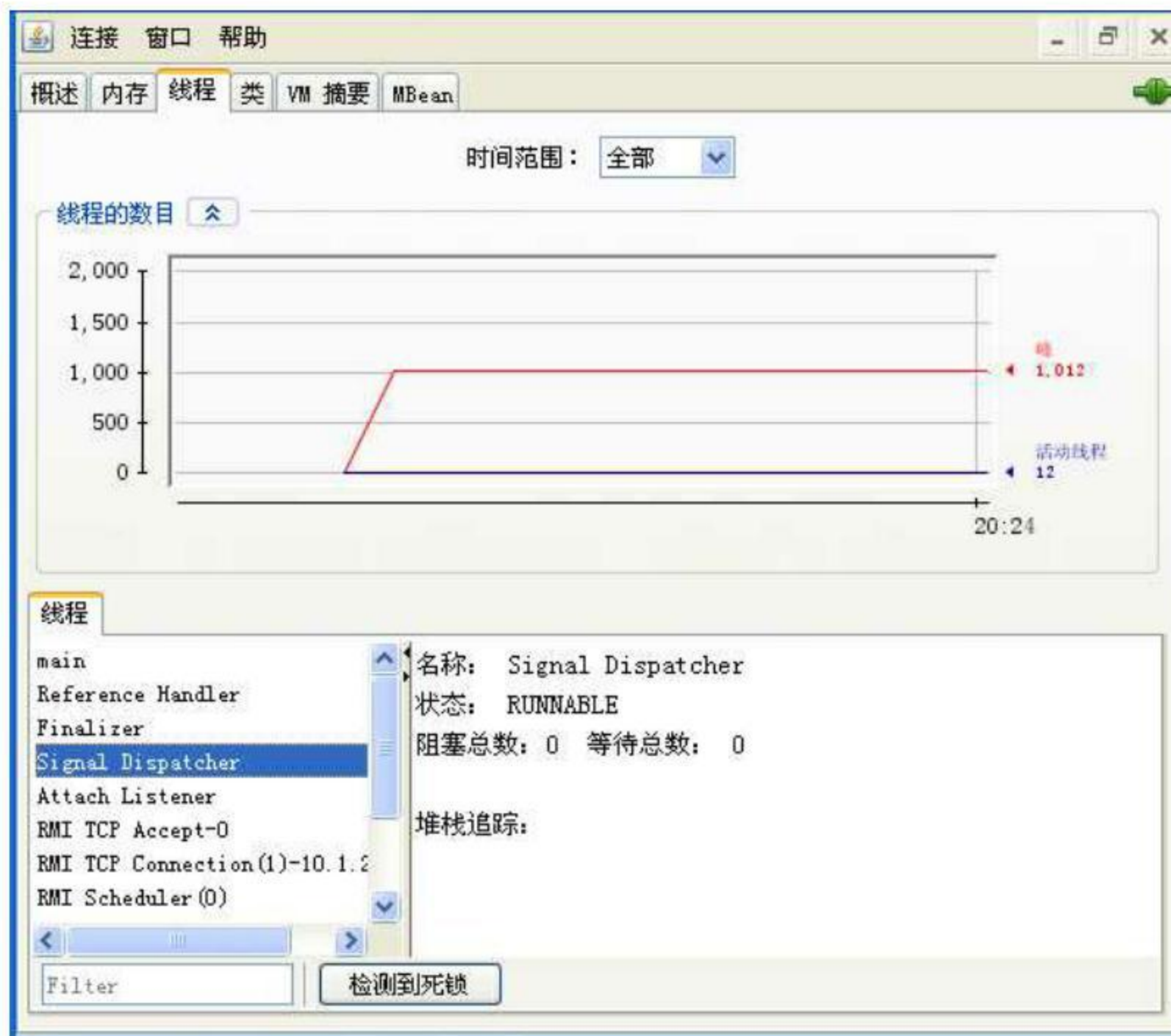
图 3.25 JConsole 查看线程状态
