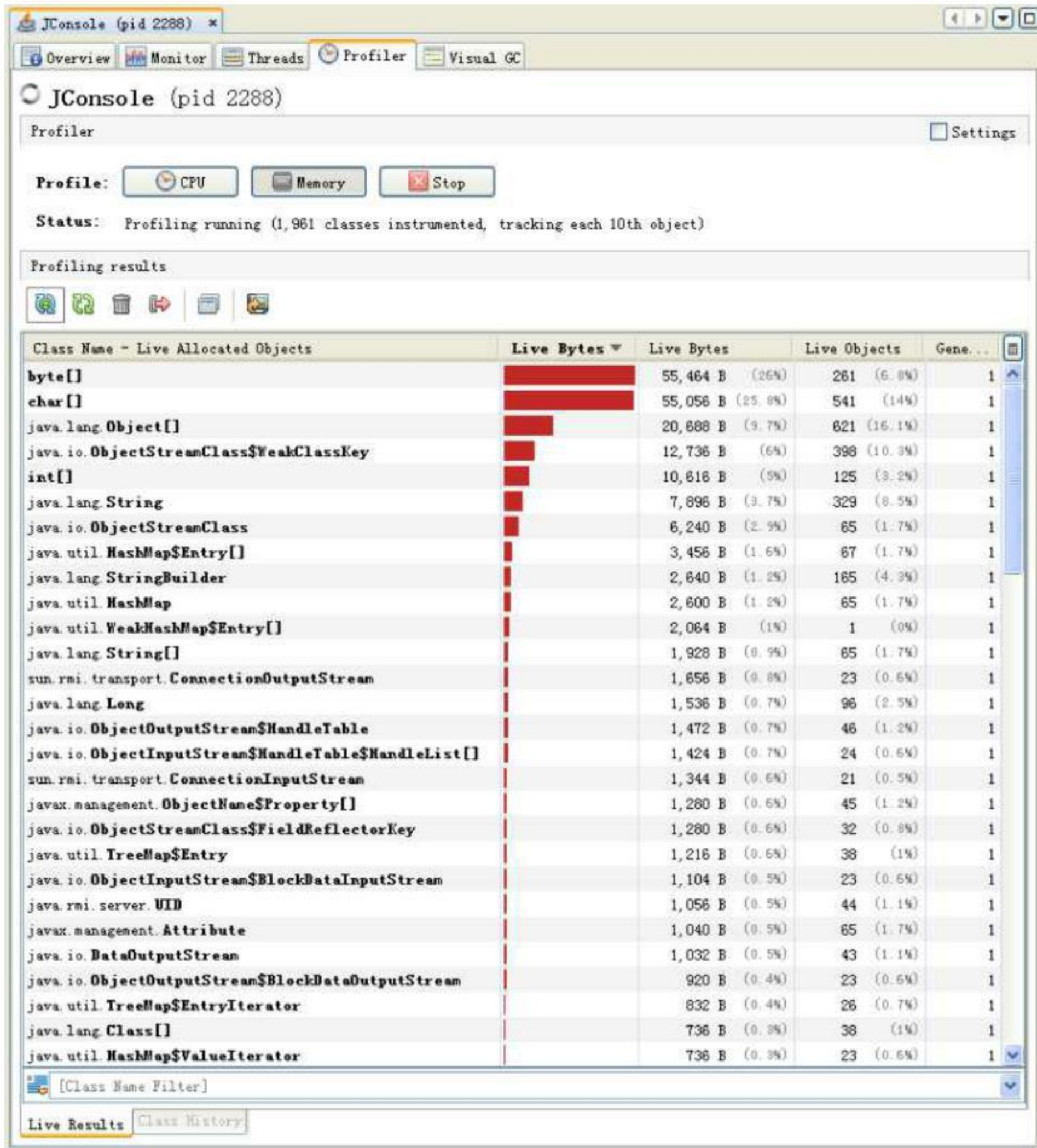
图 3.20 JVisualVM Memory Profiler 图示
