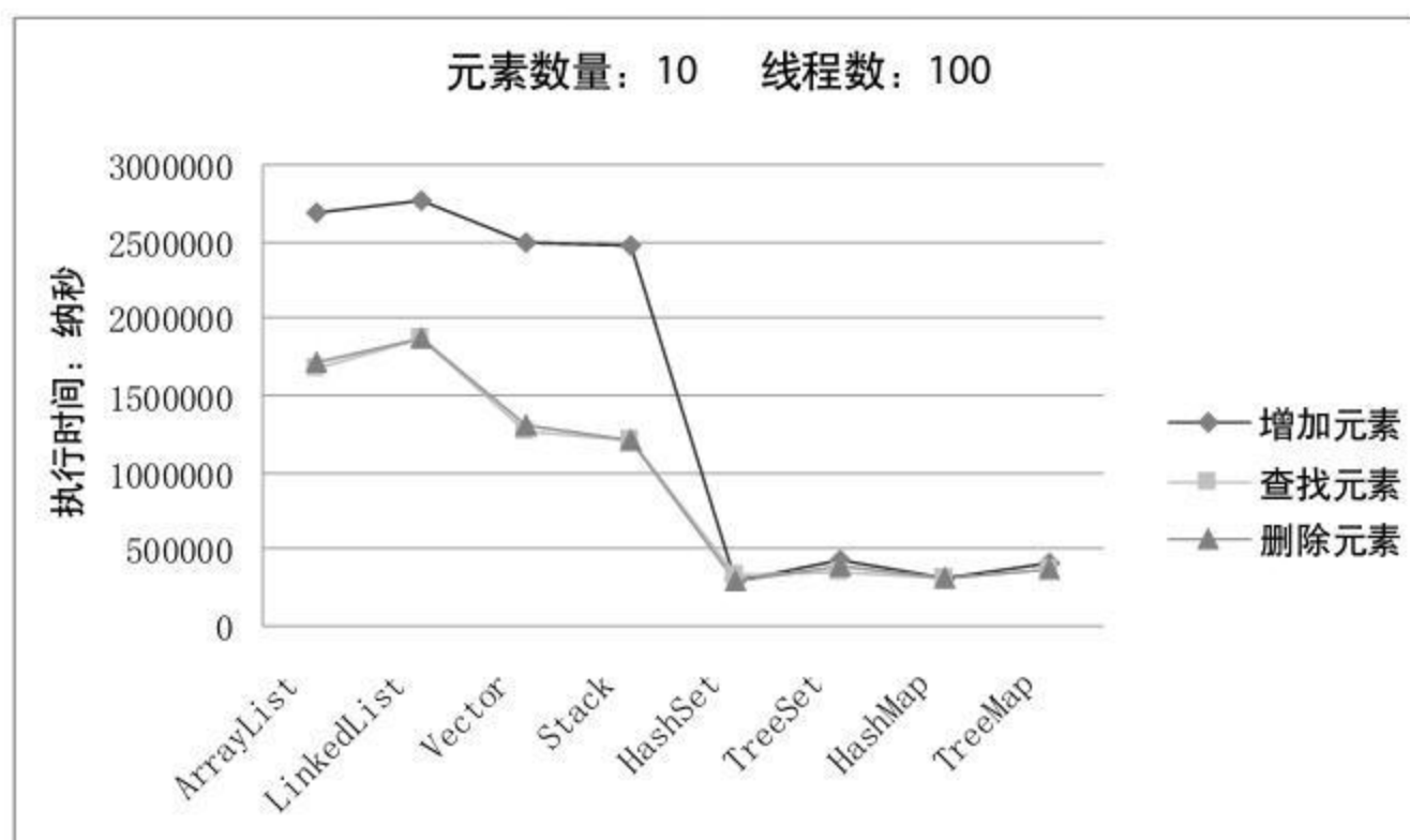
图 4.7 线程数：100，元素数量：10 时的运行结果对比
