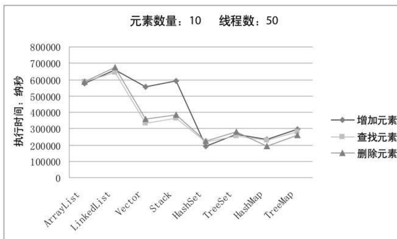
图 4.6 线程数：50，元素数量：10 时的运行结果对比
