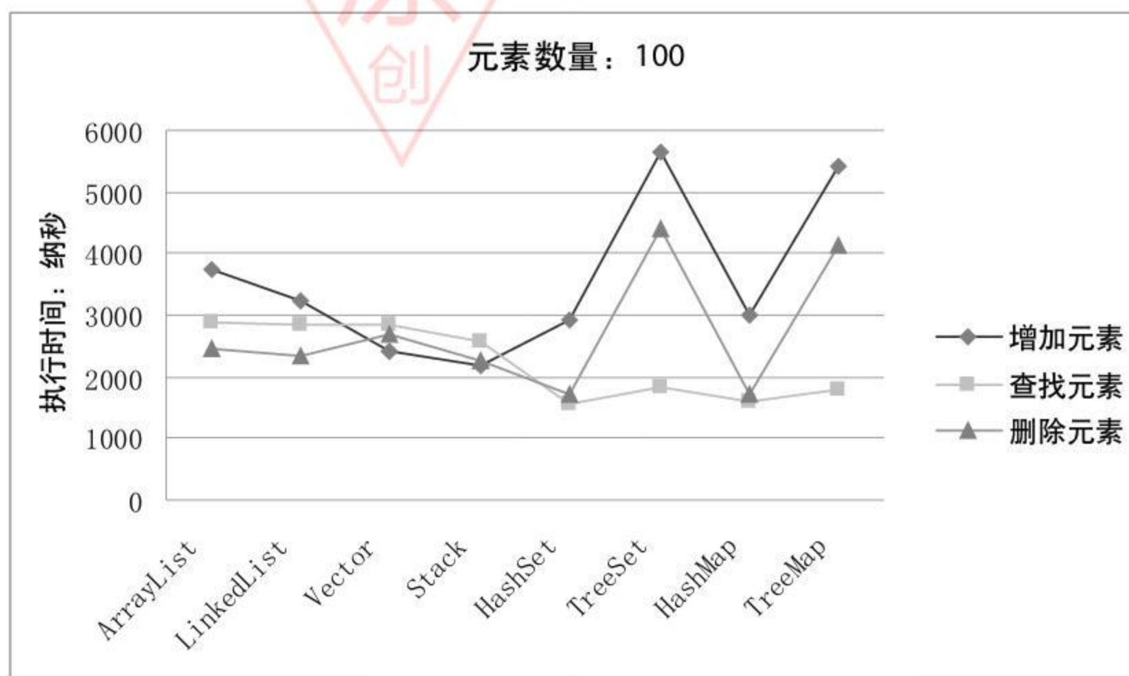
图 4.2 单线程下元素数量为 100 时的运行结果对比
