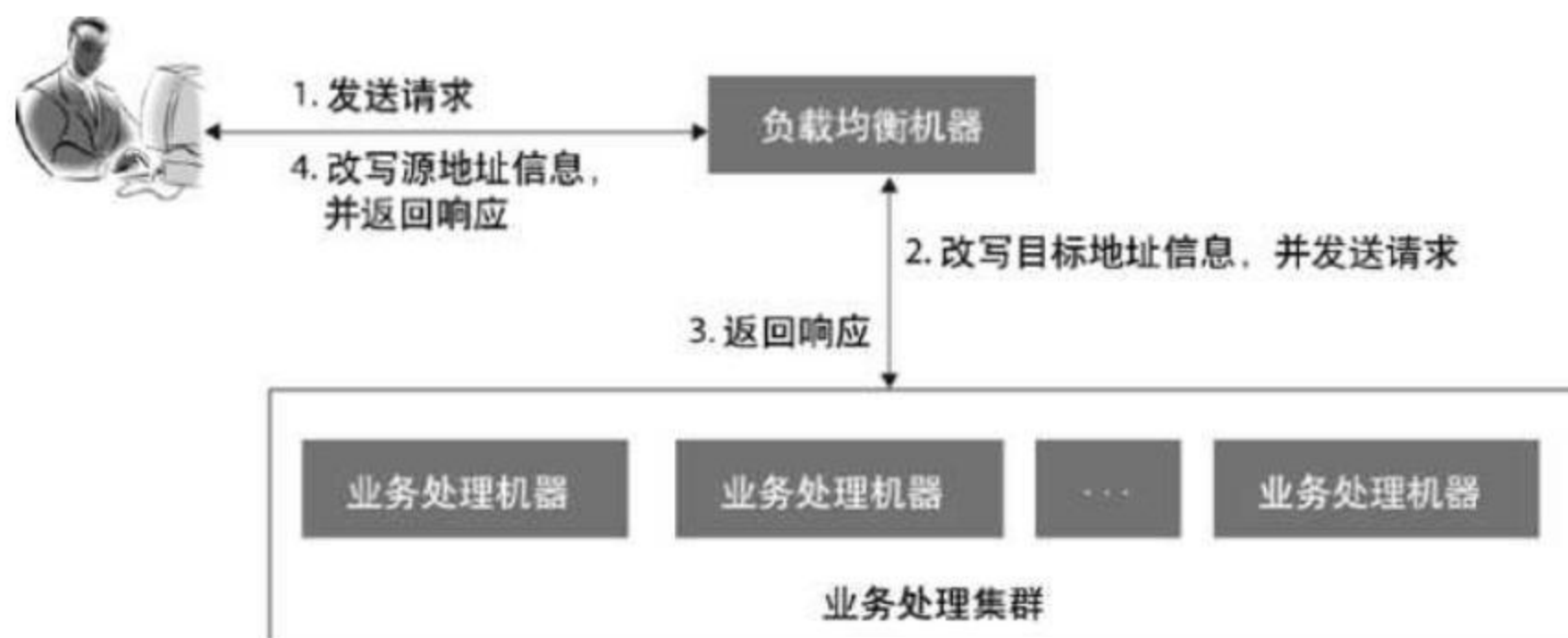
图 6.2 NAT 方式时的响应返回
