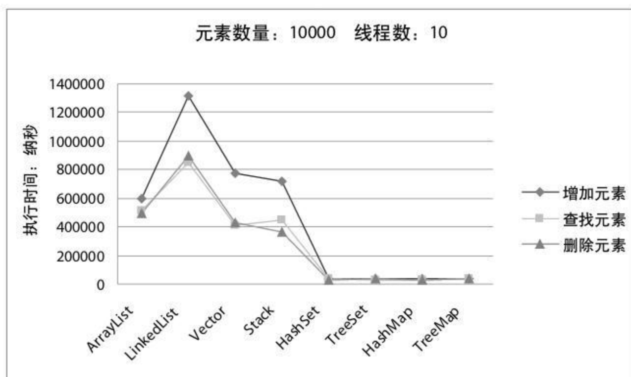
图 4.14 线程数: 10, 元素数量: 10000 时的运行结果对比
