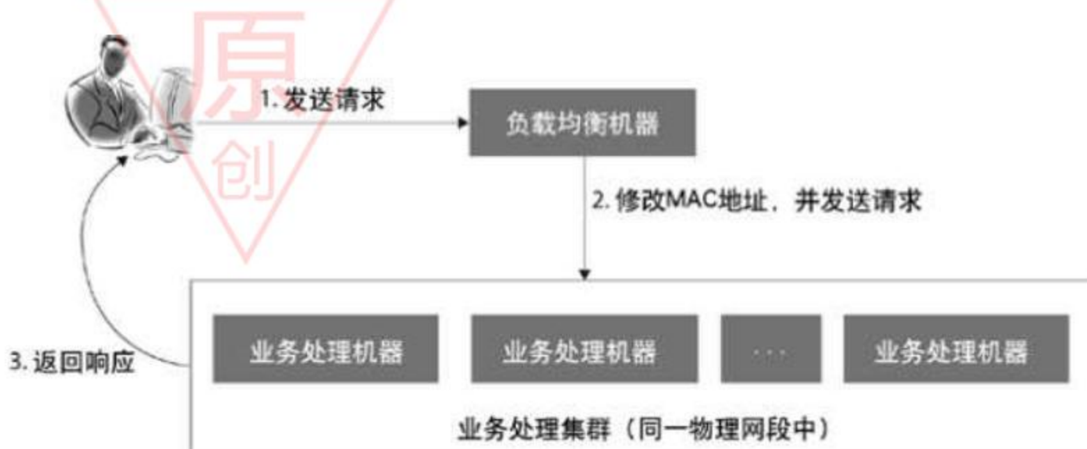
图 6.4 DSR 方式时的响应返回
