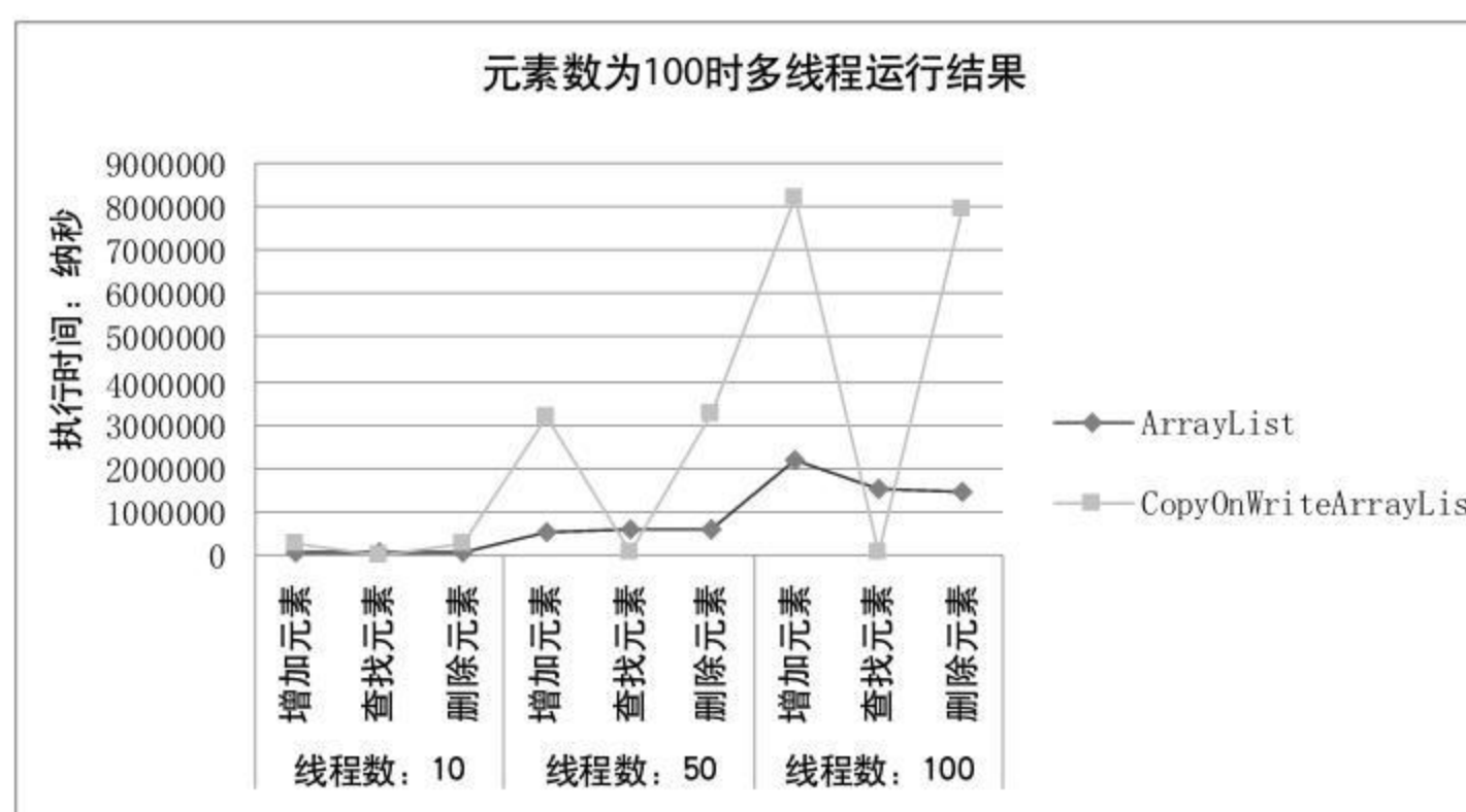
图 4.24 多线程下，元素数为 100 时 CopyOnWriteArrayList 和 ArrayList 的对比
