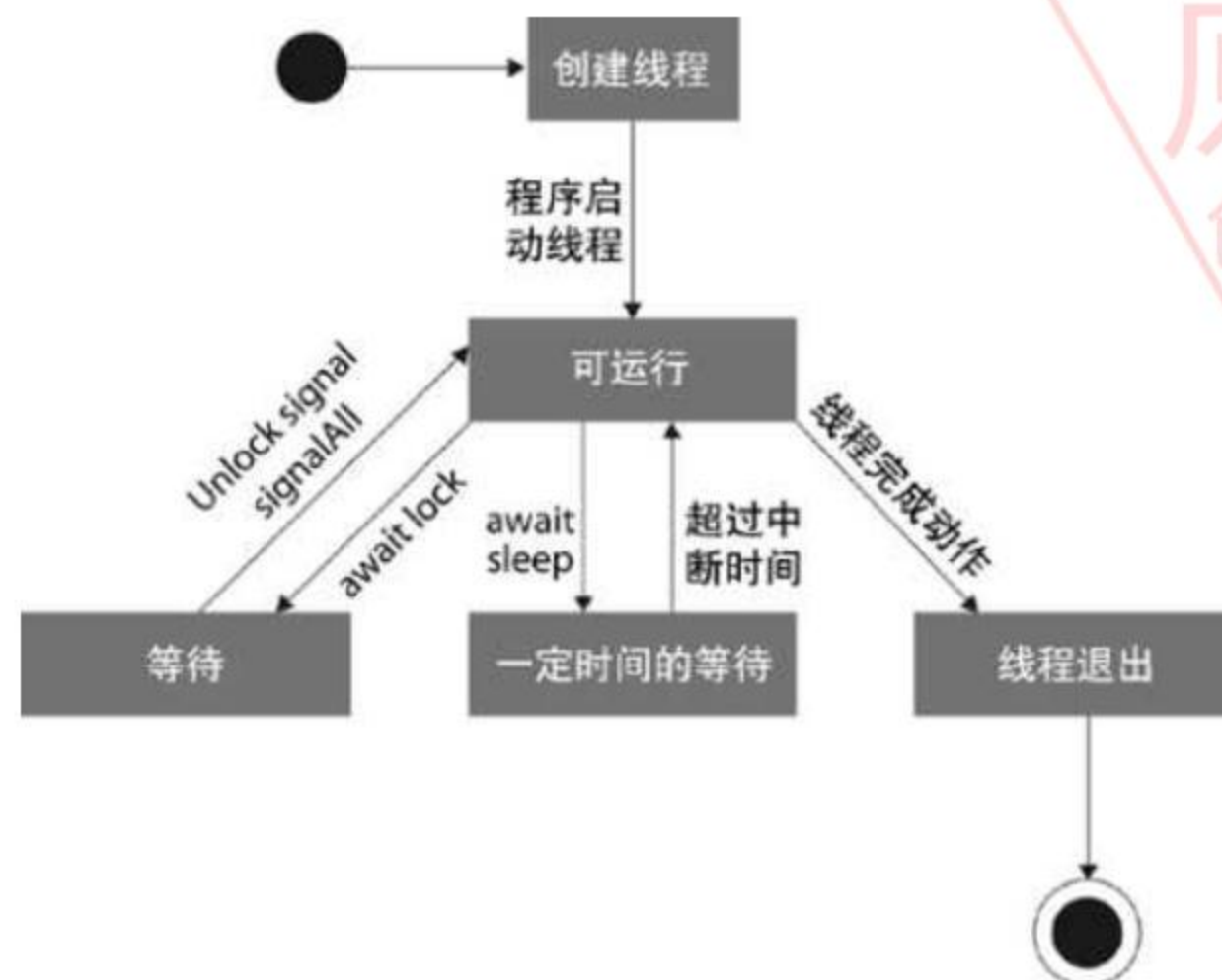
图 3.24 JVM 线程状态转换
