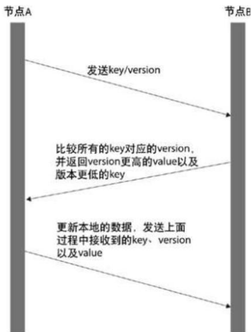
图 6.5 Gossip 模型
