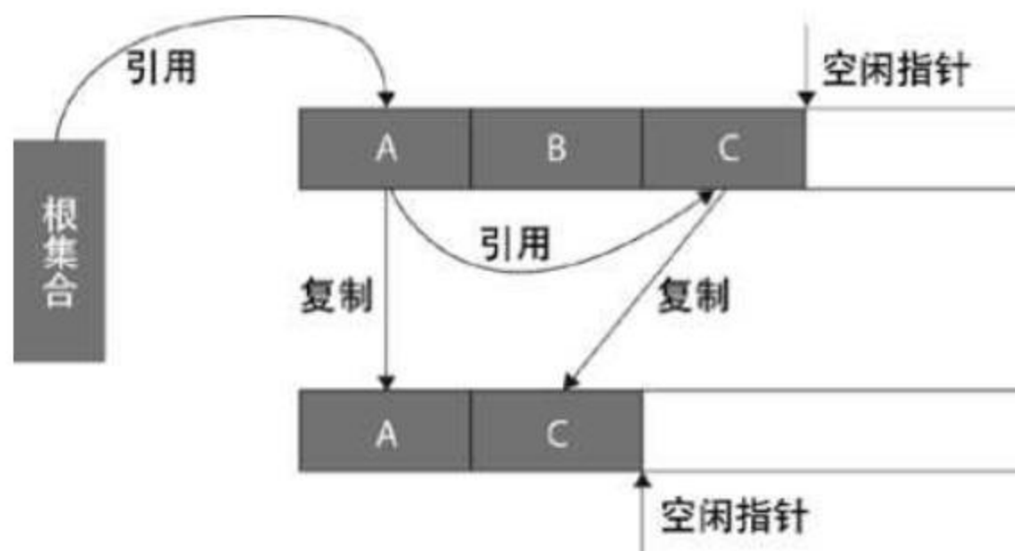
图 3.10 复制算法
