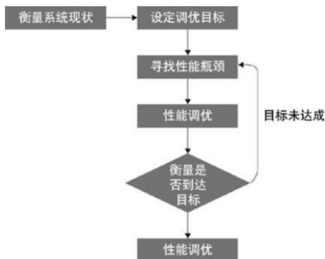
图 5.1 调优步骤
