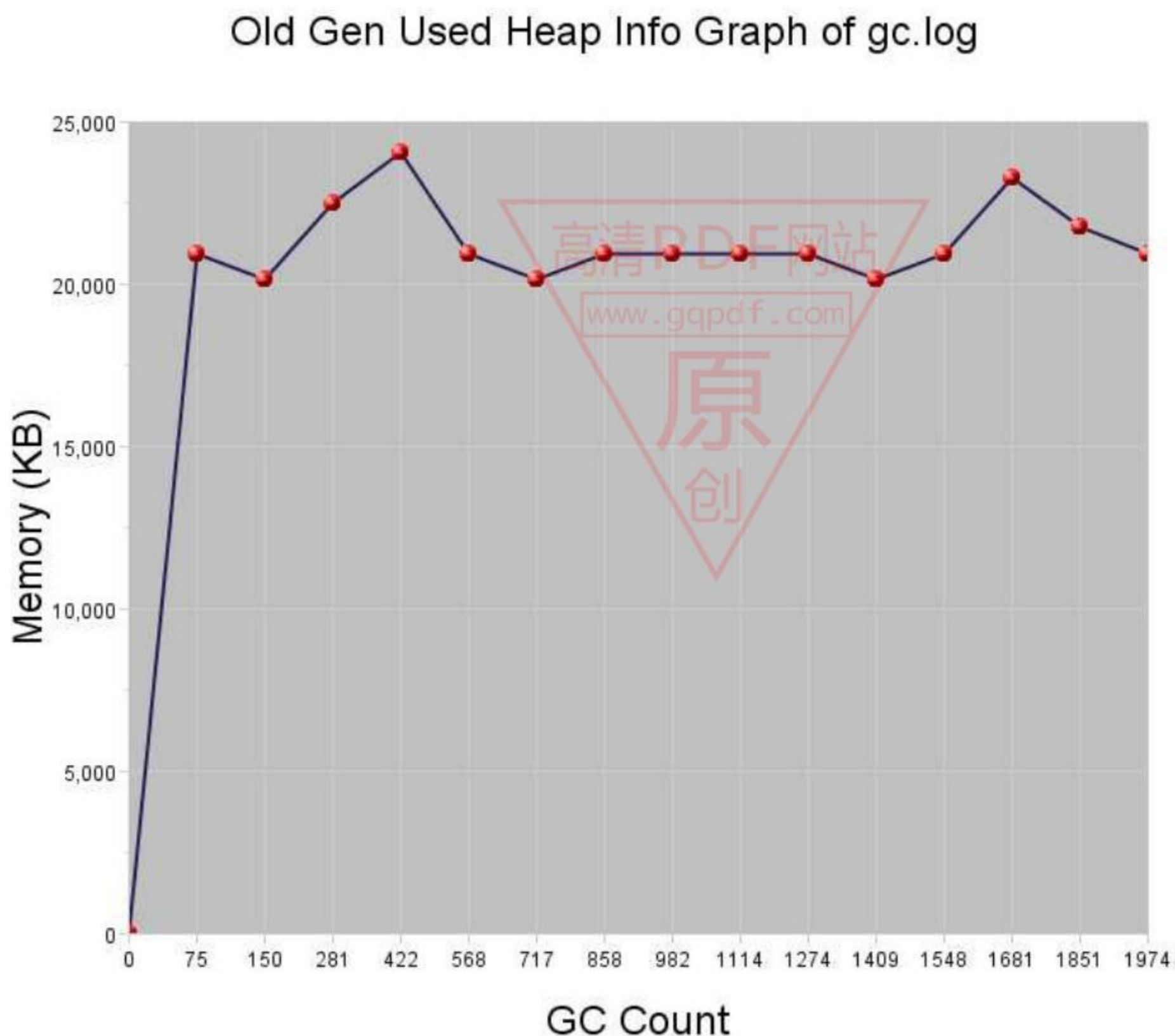
图 3.17 GCPortal 示例
