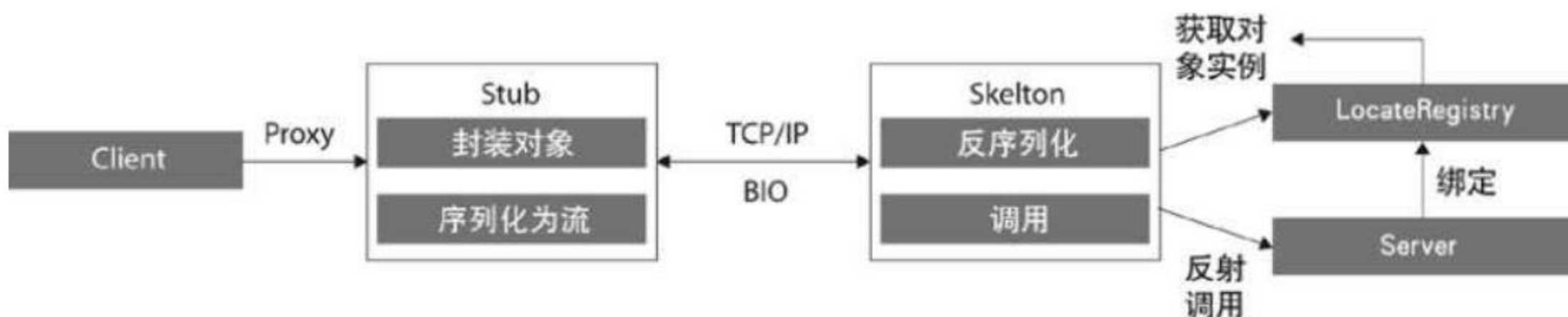
图 1.1 RMI 机制
