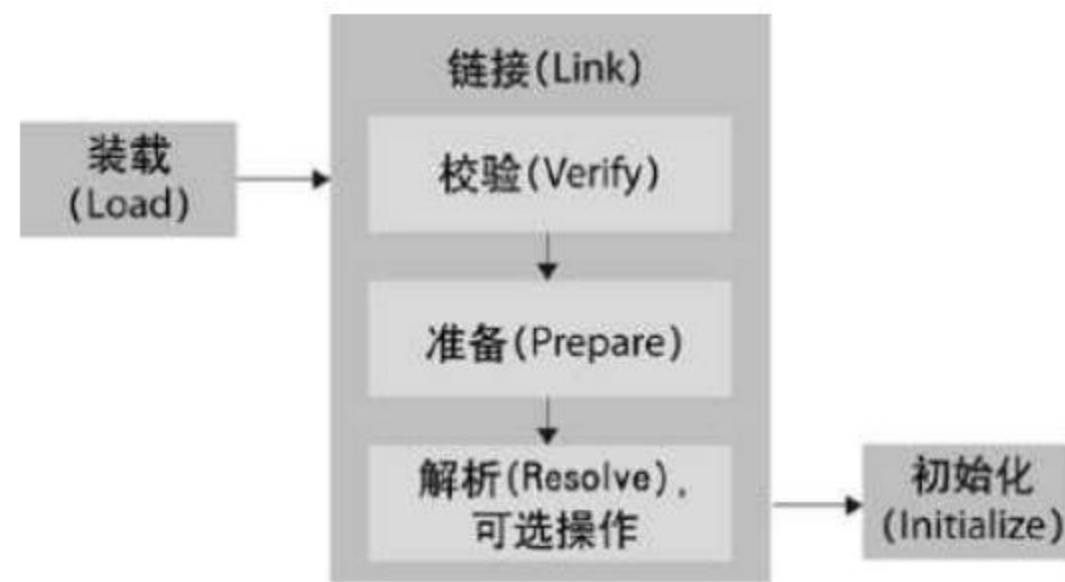
图 3.3 类加载过程
