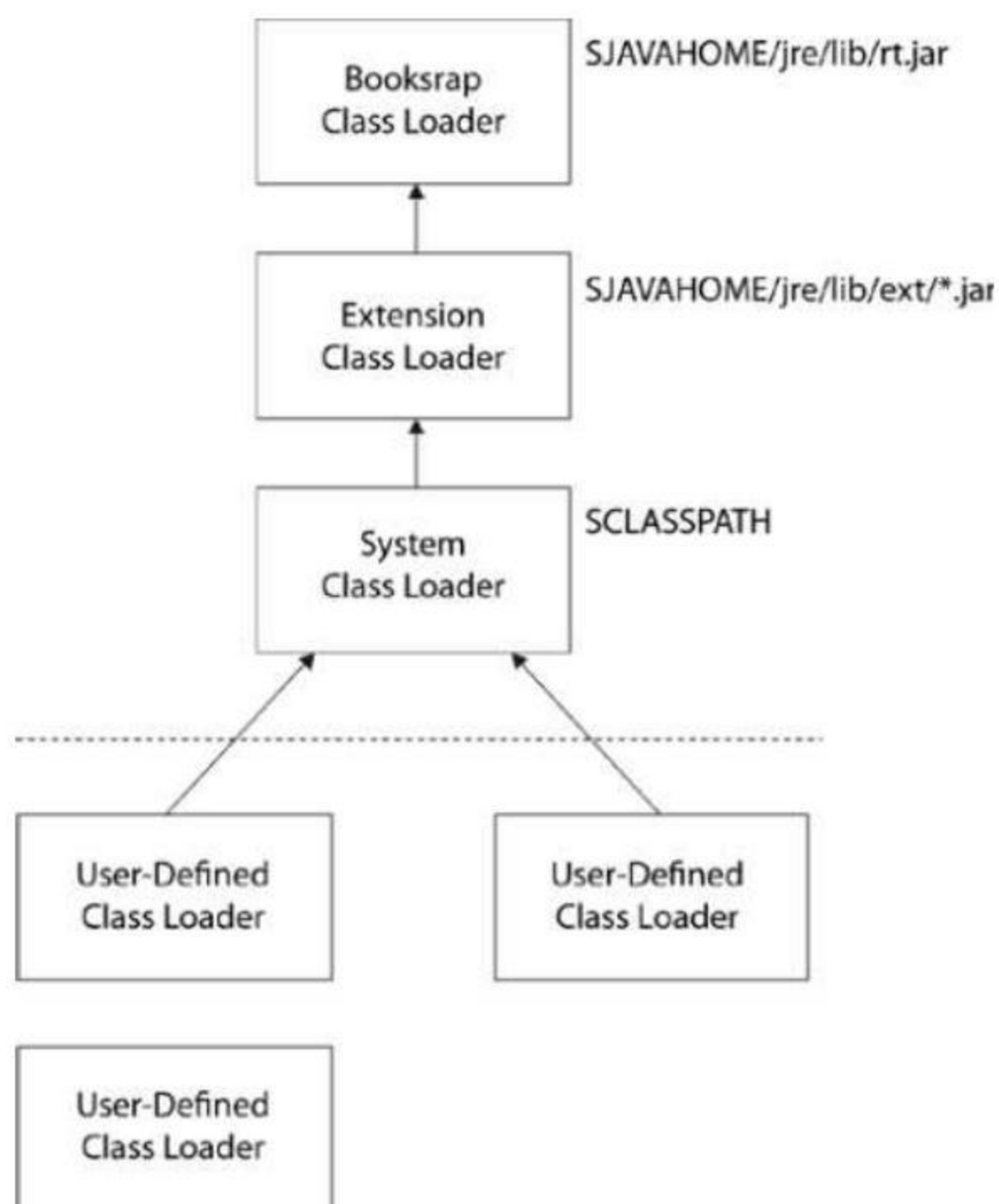
图 3.4 Sun JDK ClassLoader 继承关系
