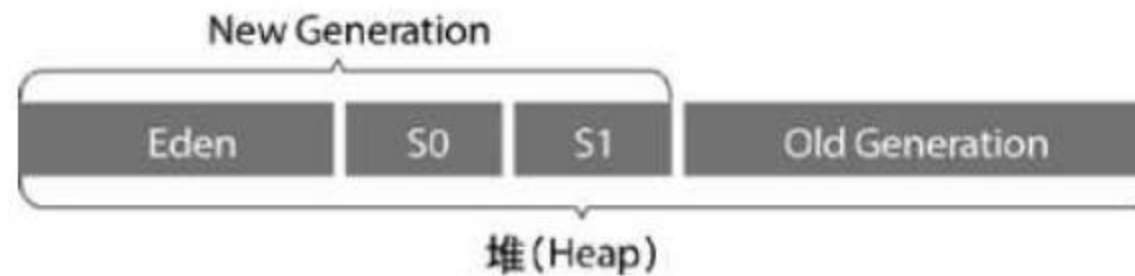
图 3.8 Sun JDK 堆的分代
