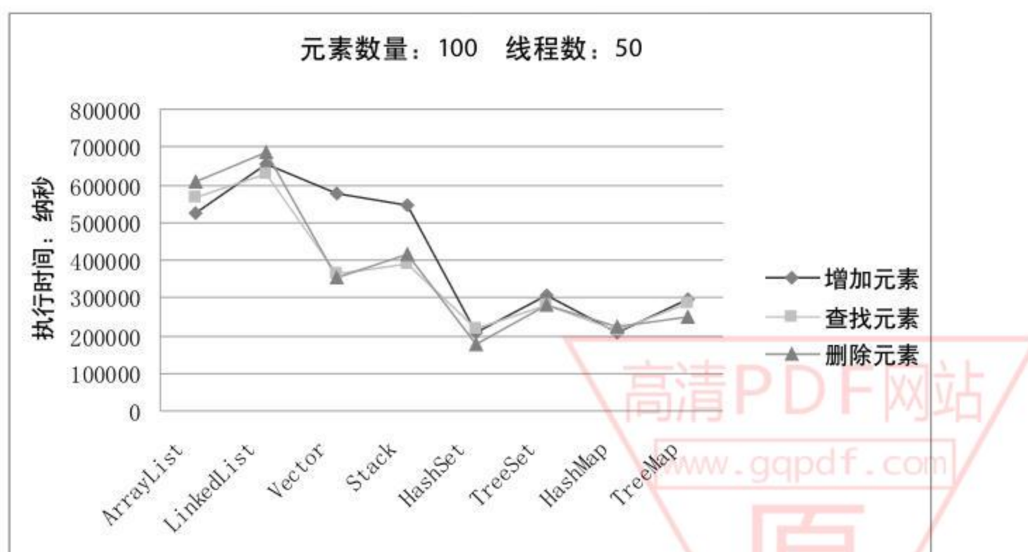
图 4.9 线程数: 50, 元素数量: 100 时的运行结果对比
