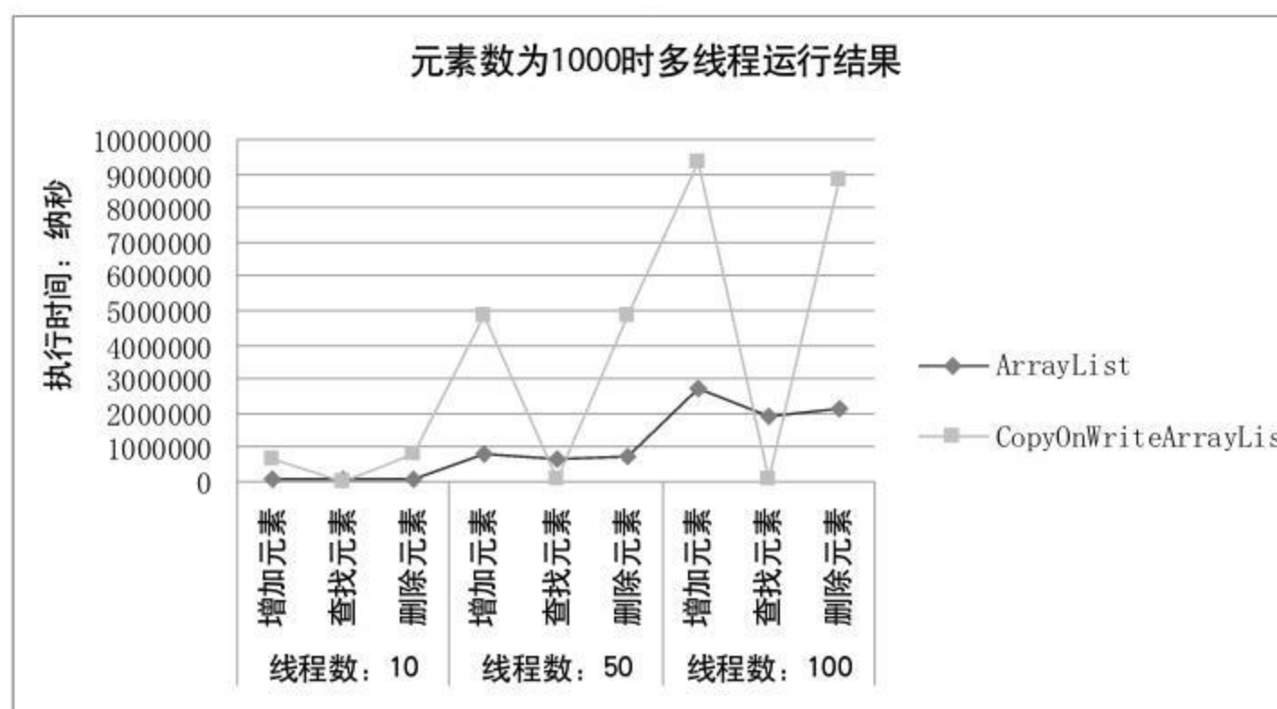
图 4.25 多线程下，元素数为 1000 时 CopyOnWriteArrayLis 和 ArrayList 的对比
